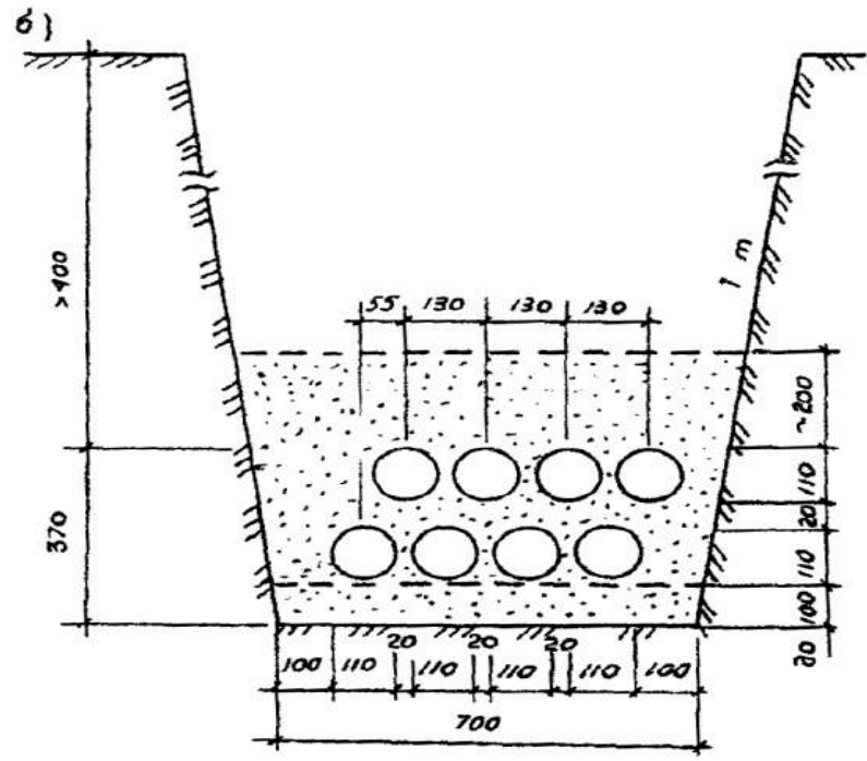
а – друг над другом; б – со смещением Рисунок 1 – Схемы расположения каналов связи из труб ТПЭ-КЭС в блоках
